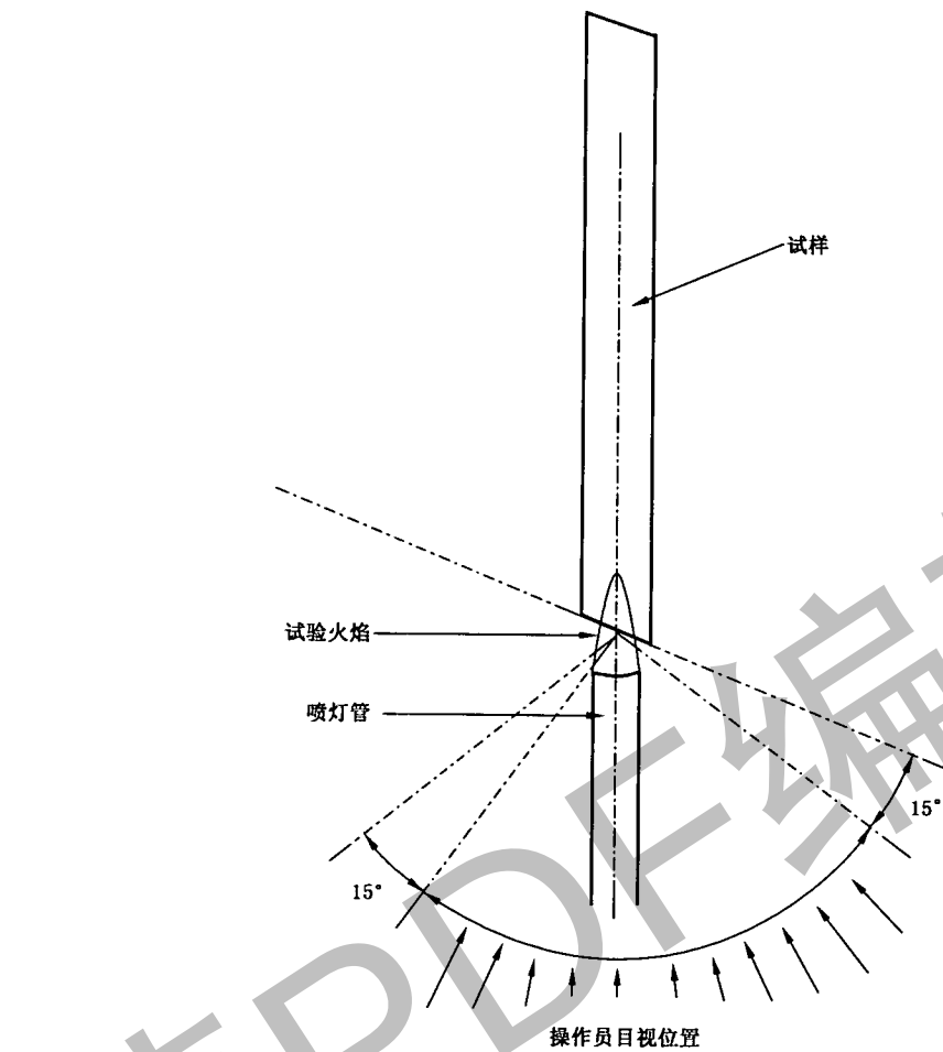
图 6 喷灯/操作员/试样的排列方位
