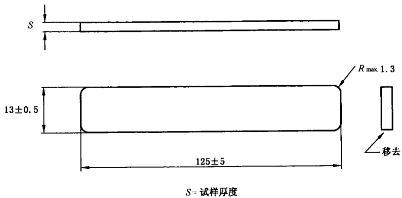
图 4 条状试样
