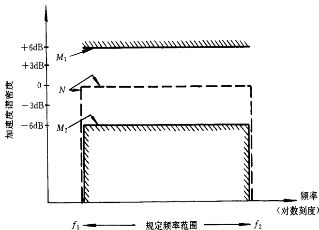
M_1 —容差上限,中再现性; M_2 —容差下限,中再现性; N —规定的加速度谱密度的标称值
