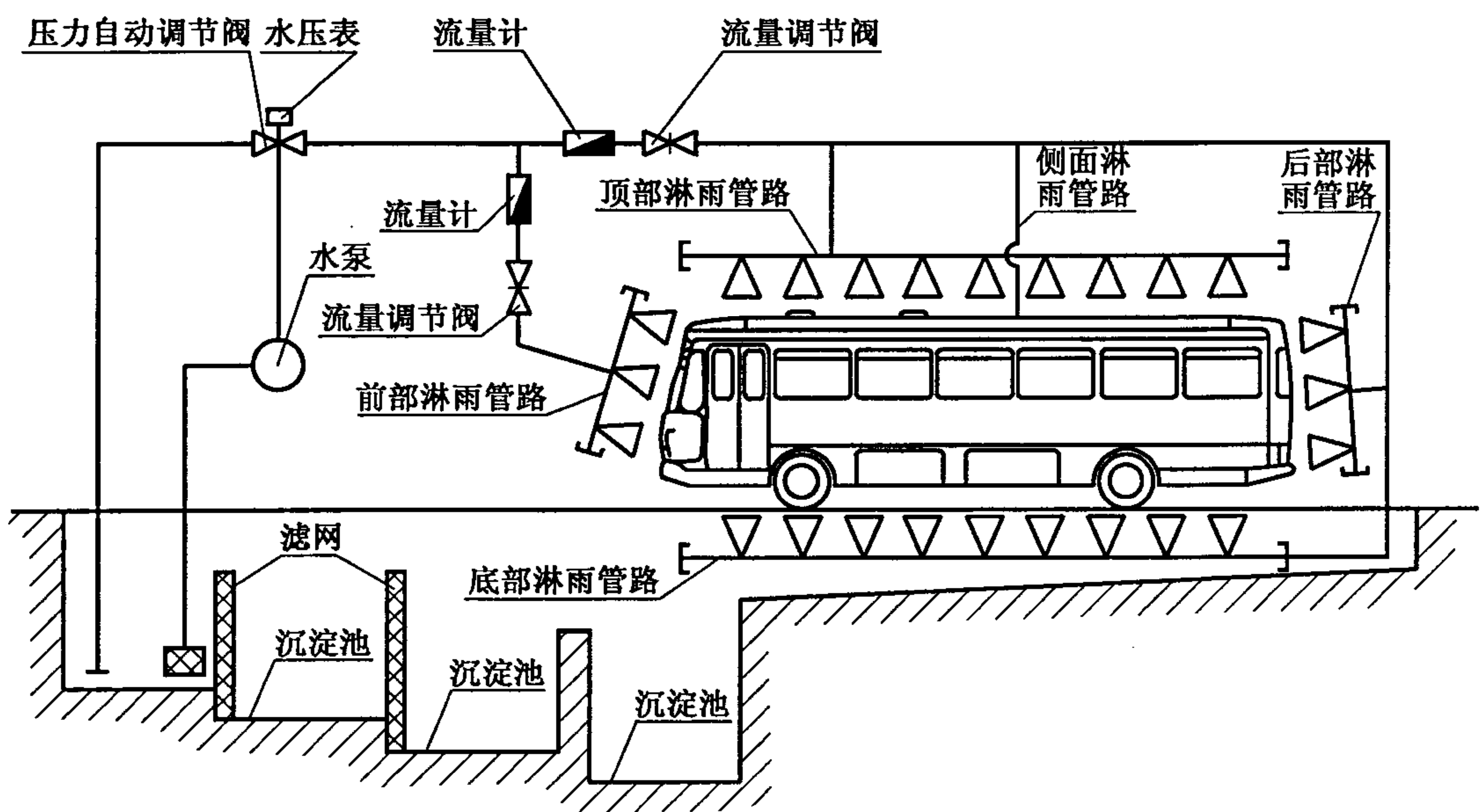
图 A.1 淋雨装置示意图
