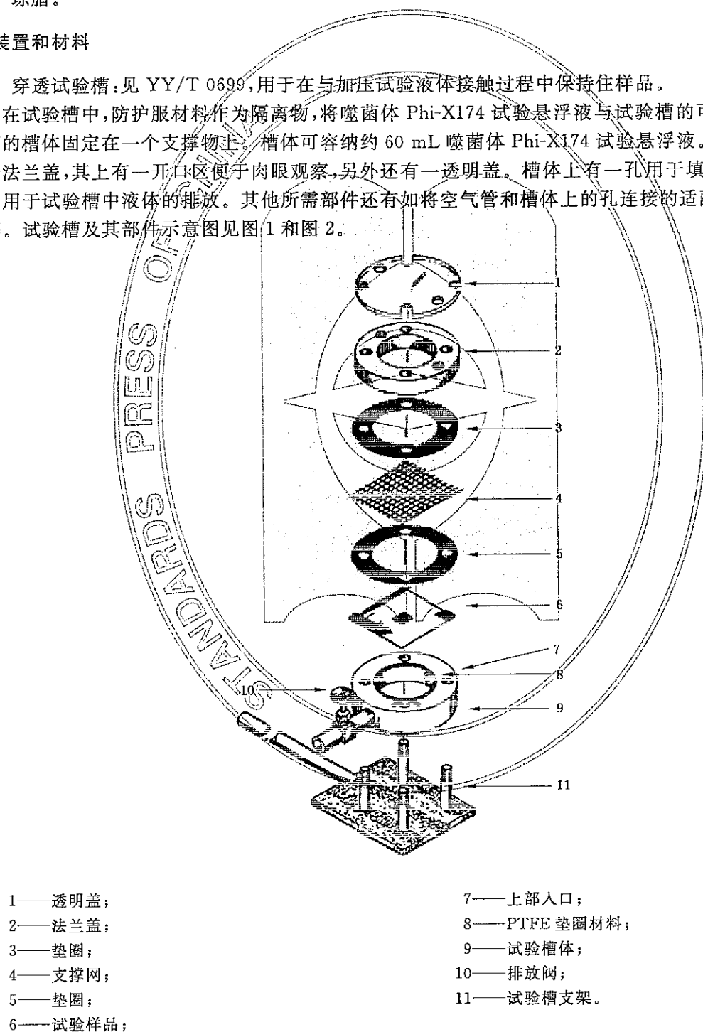
图 1 试验槽结构
