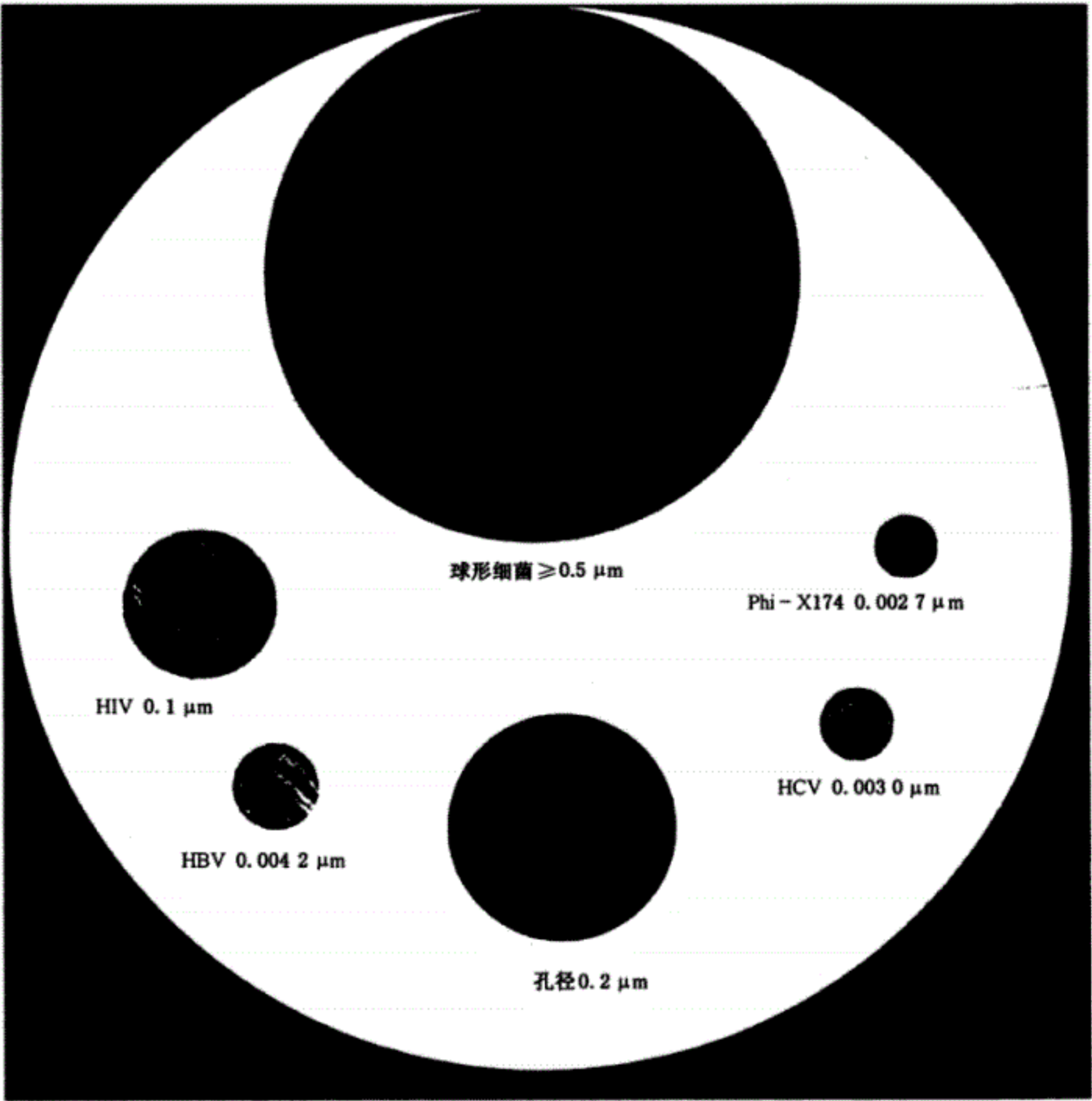
图 1 球形致病菌大小对比
