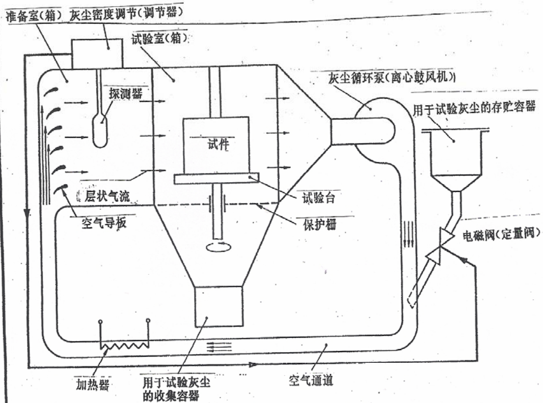
图2 为证明对灰尘防护效果的试验装置; 外来物防护级别 5K级和6K级(图例用于具有水平灰气流方向的灰室)
