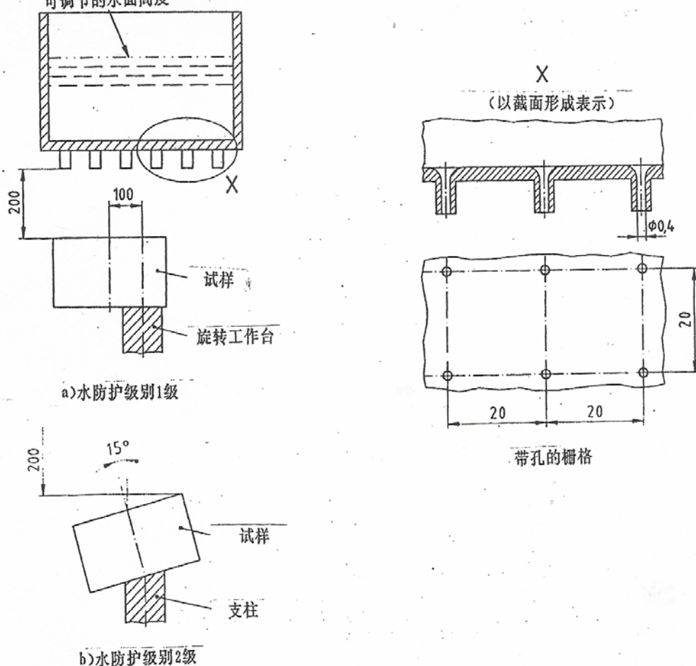
图3: 用来证明对垂直落下之水滴的防护效果的试验装置 (水滴计); 水防护级别1级和2级
