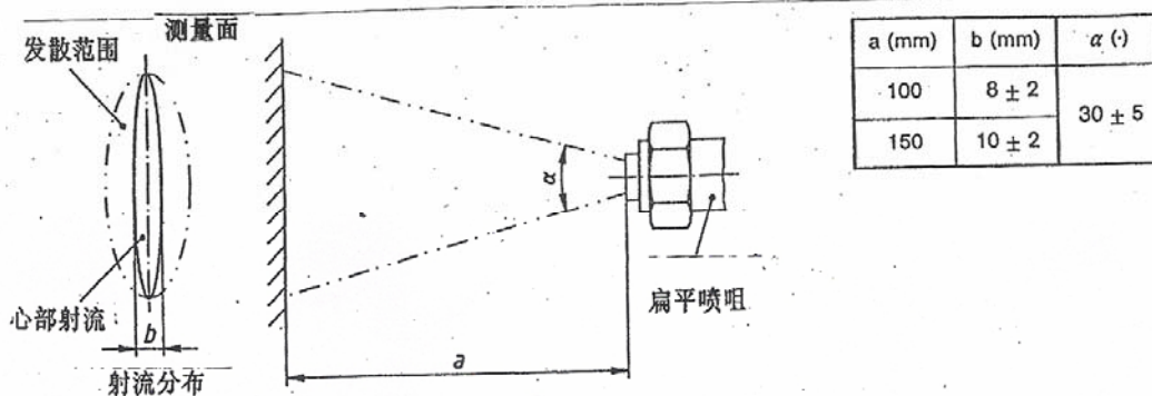
图7: 用来证明对高压/蒸汽喷射清洗之防护效果的试验装置 及其扁平喷嘴和射流分布; 9K级水防护
